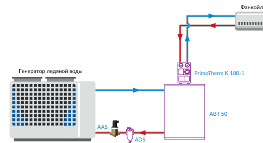
Рис. 3. Примеры систем с сепаратором воздуха AAS
