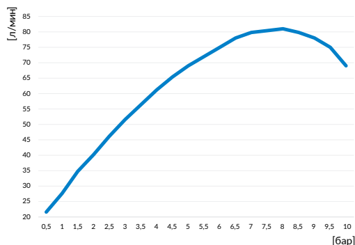
Рис. 7. Характеристики производительности отвода воздуха
