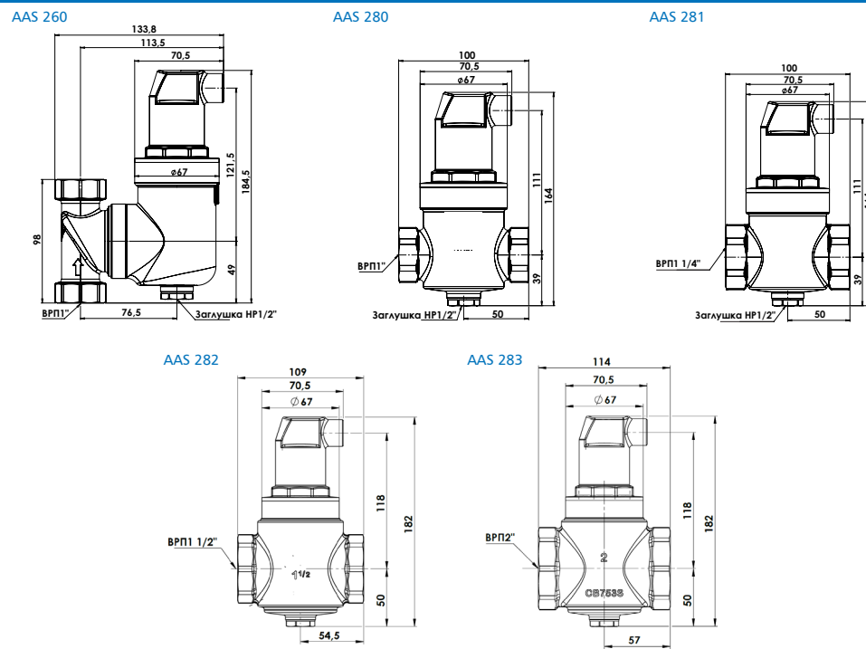
Рис. 2. Размеры сепараторов воздуха AAS
