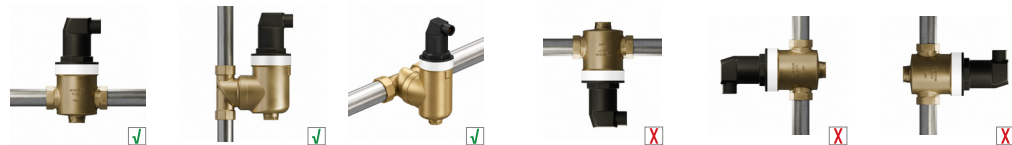
Рис. 4. Допустимое монтажное положение сепаратора воздуха AAS
