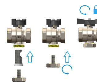
Rys. 9. Schemat złożenia zaworu kulowego BFV
