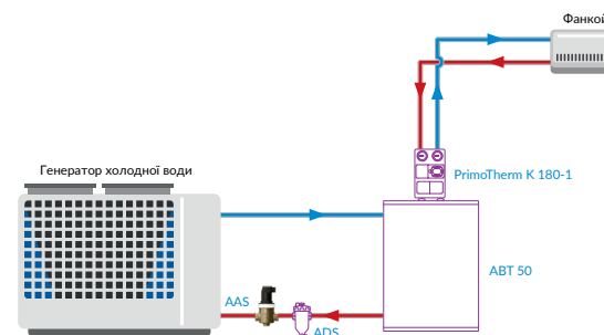
Рис. 3. Приклади систем із сепаратором повітря AAS
