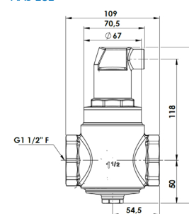
Рис. 2. Розміри сепараторів повітря AAS
