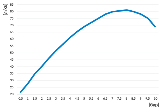
Рис. 7. Характеристики продуктивності відведення повітря
