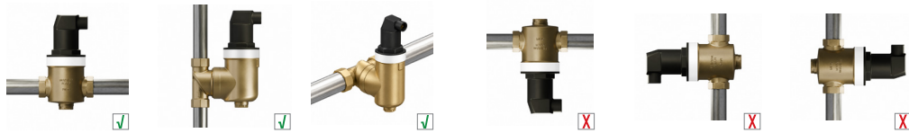
Рис. 4. Допустиме монтажне положення сепаратора повітря AAS
