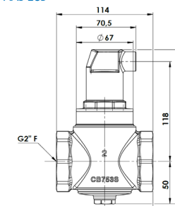
Рис. 2. Розміри сепараторів повітря AAS
