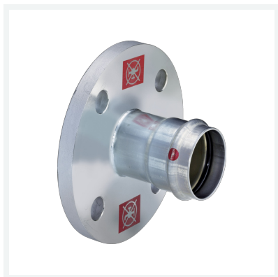
Prestabo-przejście kołnierzowe z SC-Contur nr wzoru 1159 nr kat. 643 560
