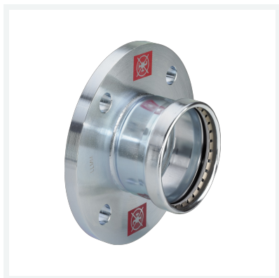
PreStabo XL-przejsie kołnierzowe z SC-Contur nr wzoru 1159.1XL nr kat. 629 939
