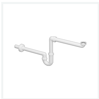
Syfon rurowy - oszczędzający miejsce wg PN-EN 274 nr wzoru 5729
