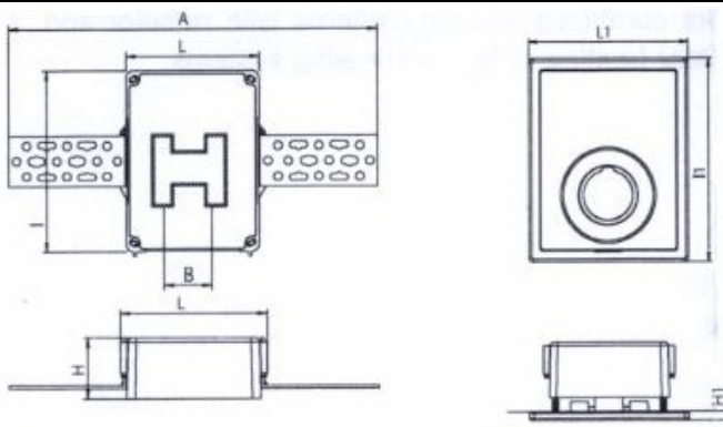
Dane techniczne ograniczników temperatury na powrocie RTL-box, głowica ukryta
