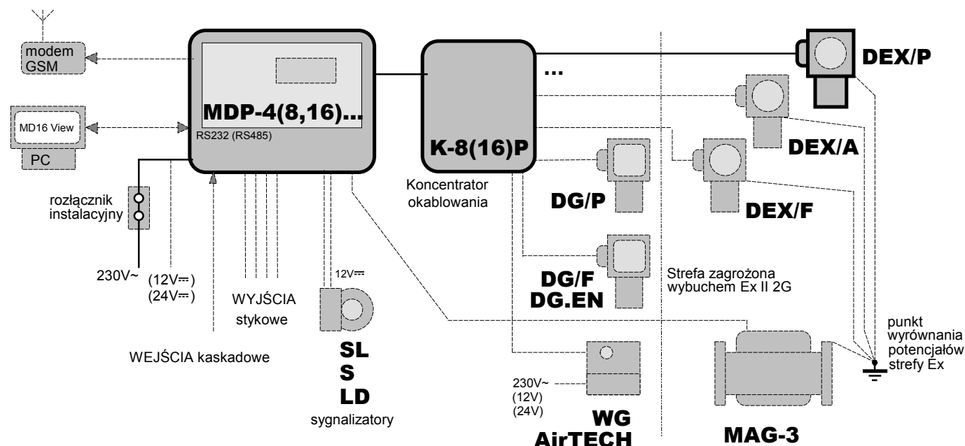
Rys.1.1. Schemat blokowy systemu
