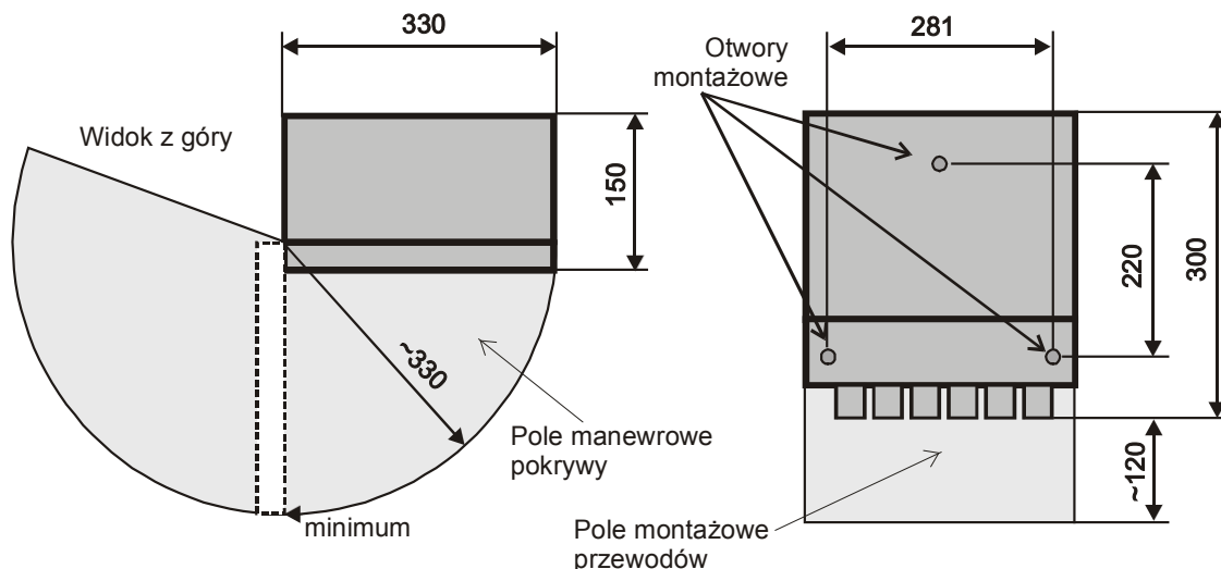
Rys.1.2. Wymagane pole montażowe
