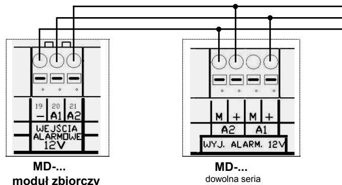
Rys.3.2.A Połączenia przewodowe różnych wariantów systemu
