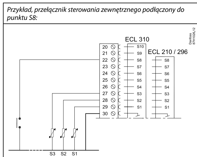
Przykład, przekaźnik sterowania zewnętrznego podłączony do punktu S8:
